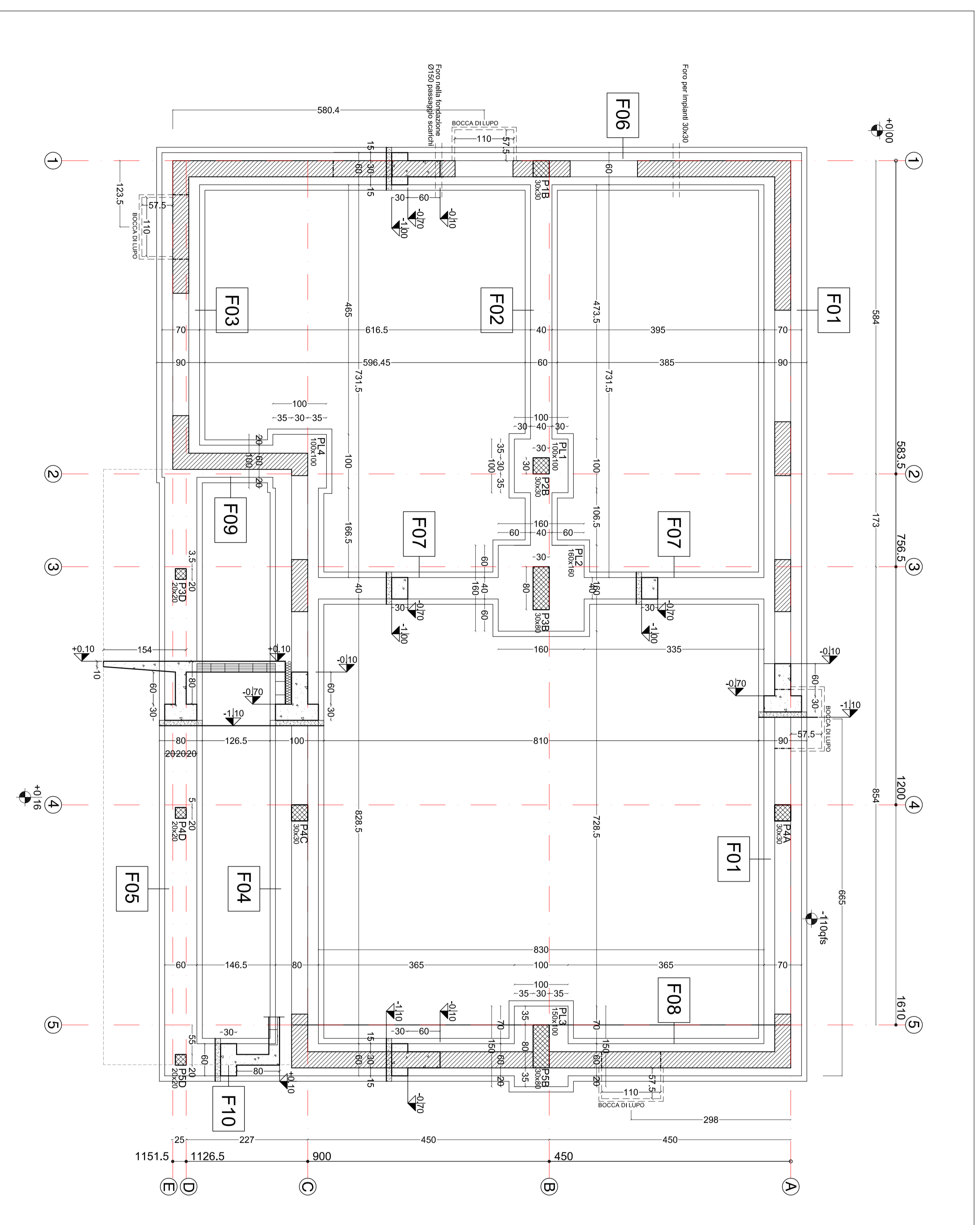
PIANTA FONDAZIONI- Scala 1:50
