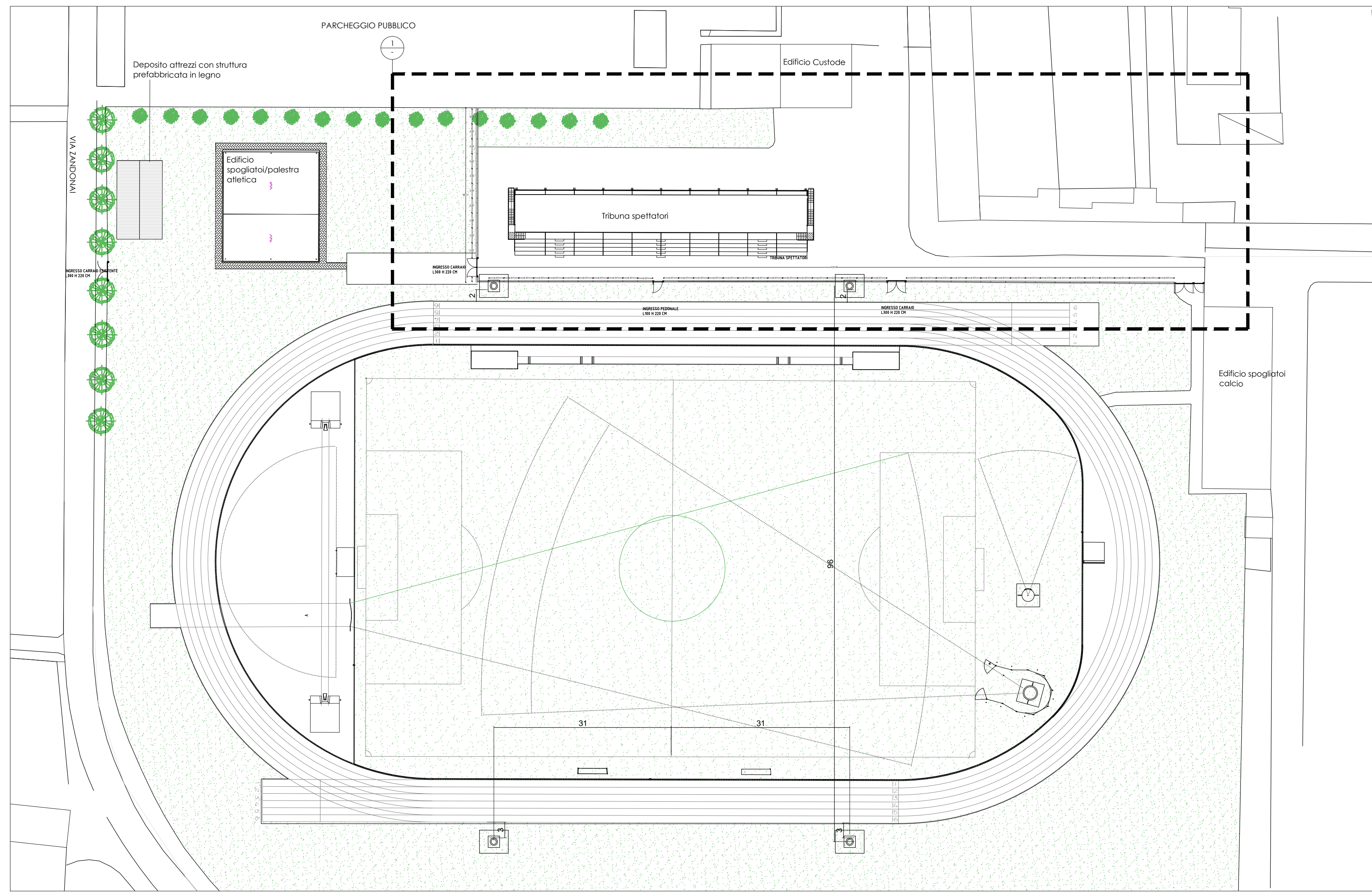
2 PROGETTO TORRI FARO E RECINZIONE PIANTA
