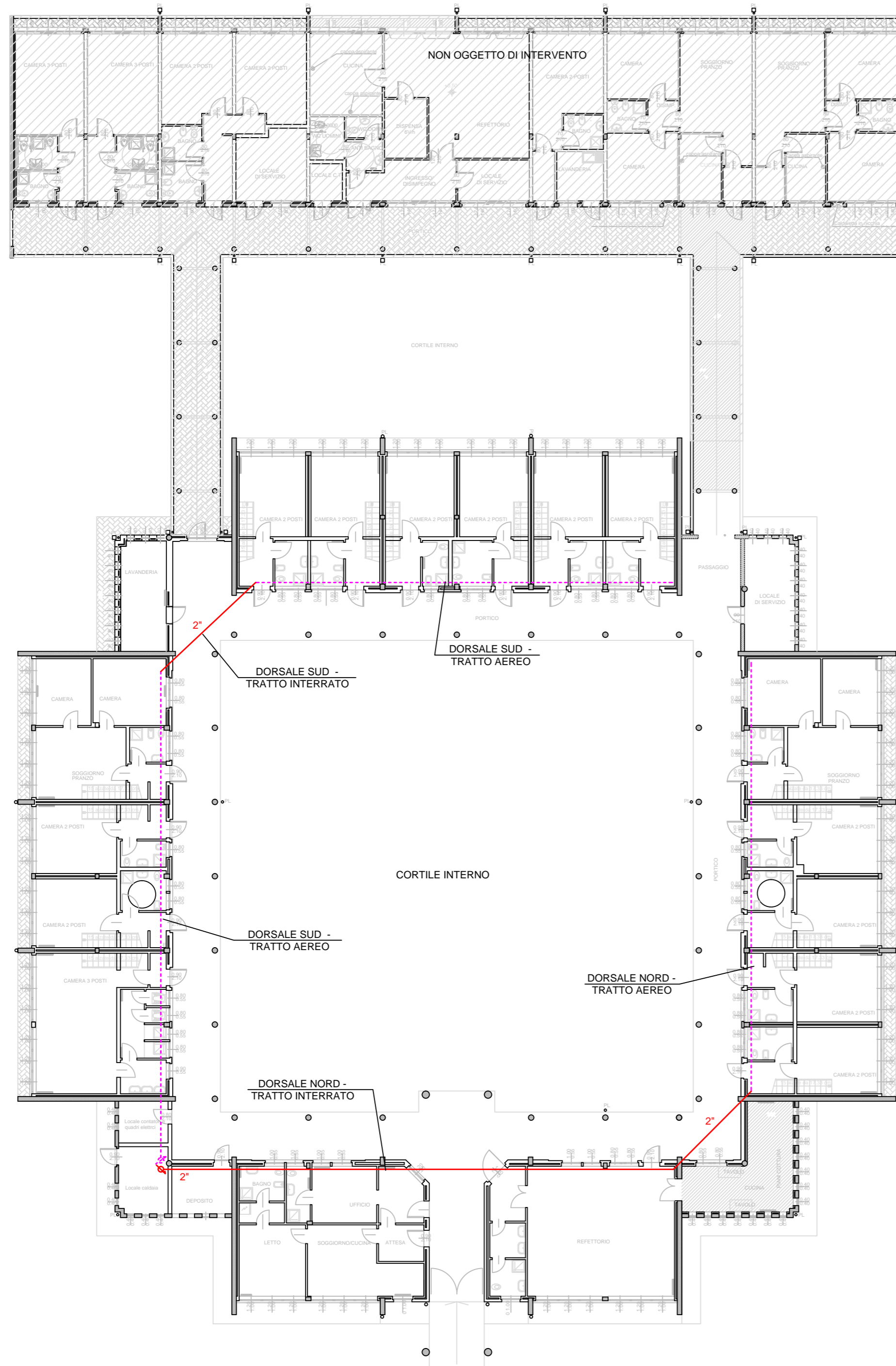
Planimetria Piano Terreno - Scala 1:200
