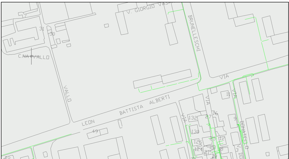
Fig. 6 - Rete telecom (estratto via Leon Battista Alberti)
