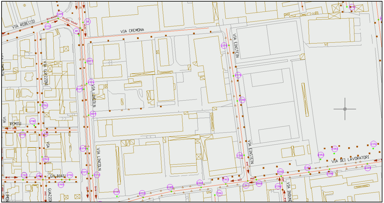
Fig. 11 - Rete fognatura (via Albert Einstein)
