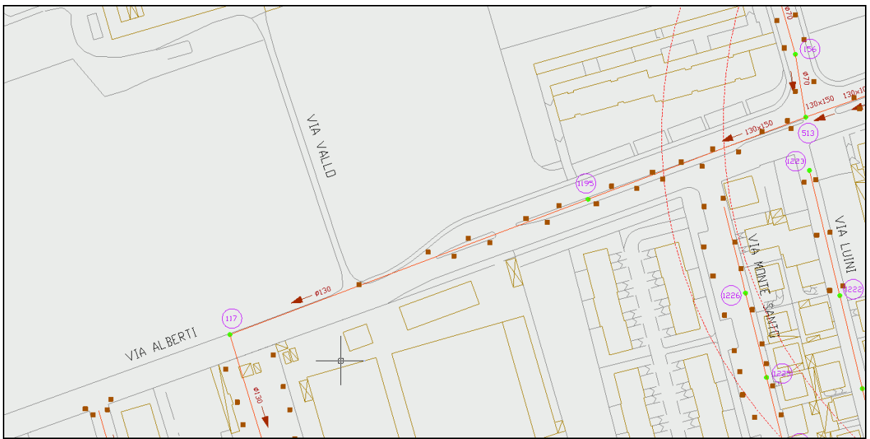
Fig. 12 - Rete fognatura (via Leon Battista Alberti)
