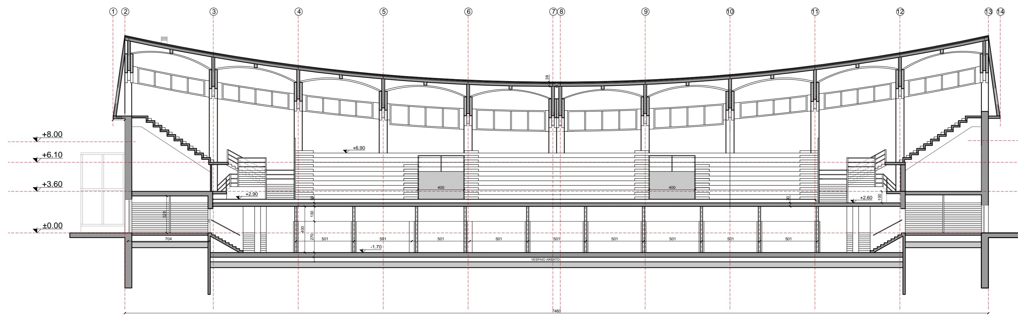
Sezione Longitudinale AA': Stato di Fatto
