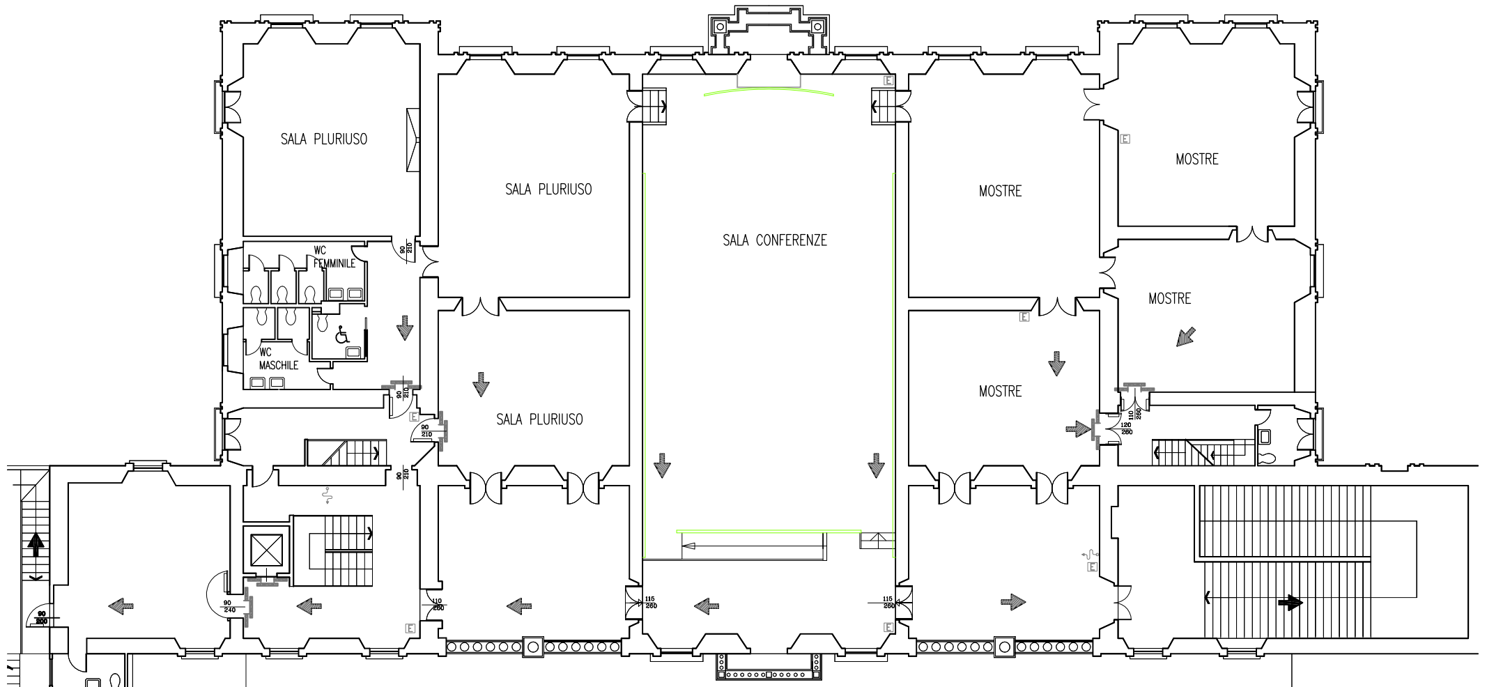
VILLA GHIRLANDA PIANTA PIANO PRIMO PARTE CENTRALE Scala 1:200
