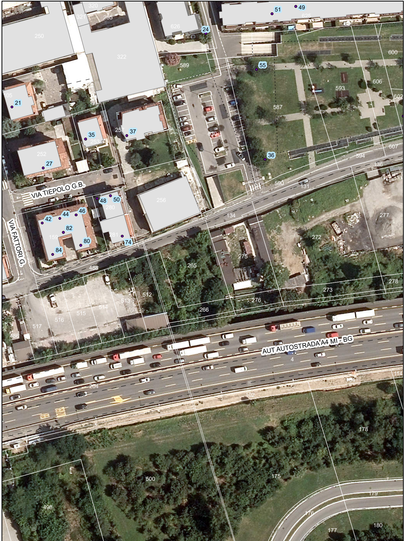
Stralcio catastale del Fg. 42 Mapp. 265 - Comune di Cinisello Balsamo Scala: 1 : 1.000
