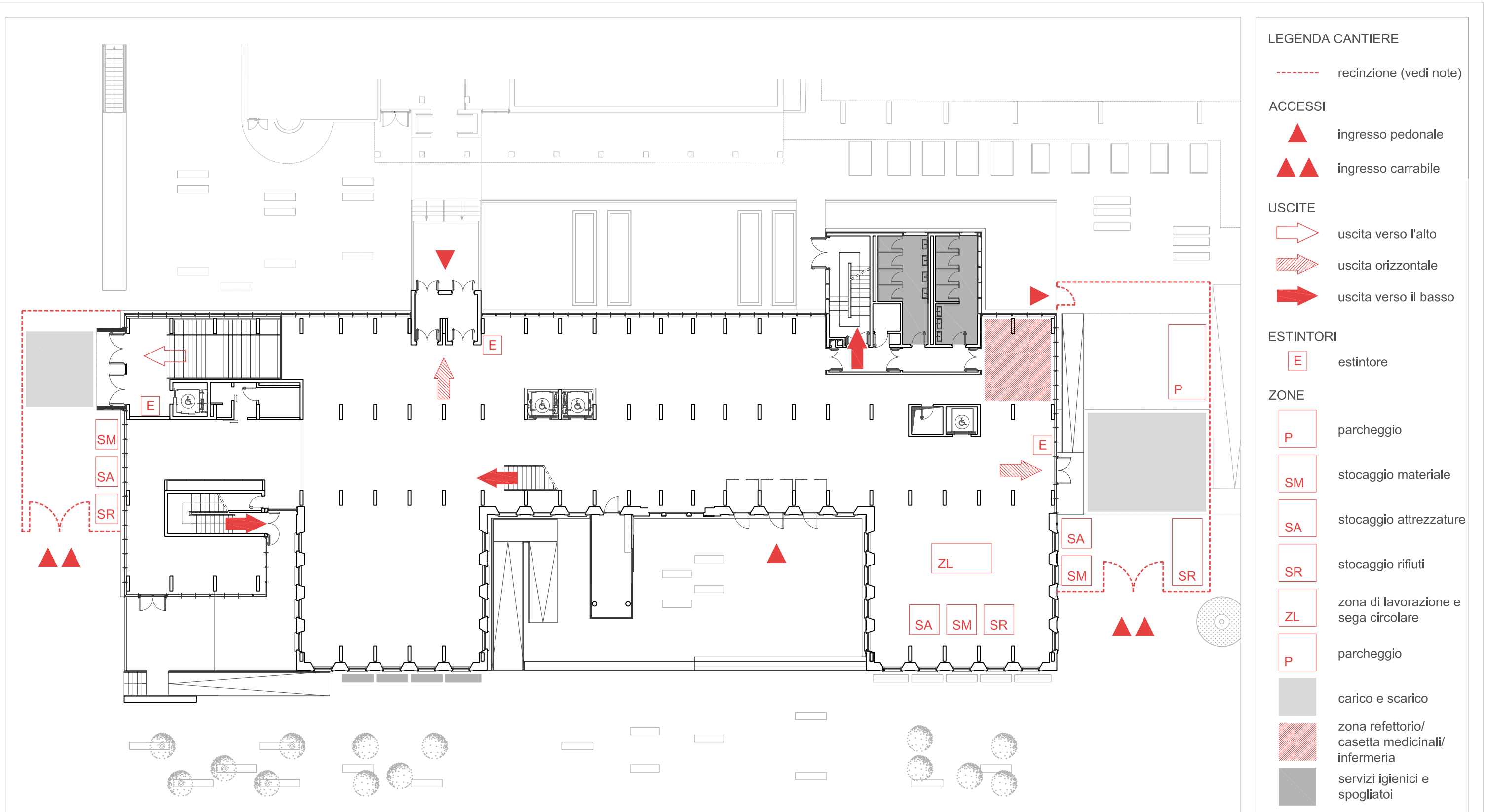
1_PANIMETRIA GENERALE DI CANTIERE, scala grafica
