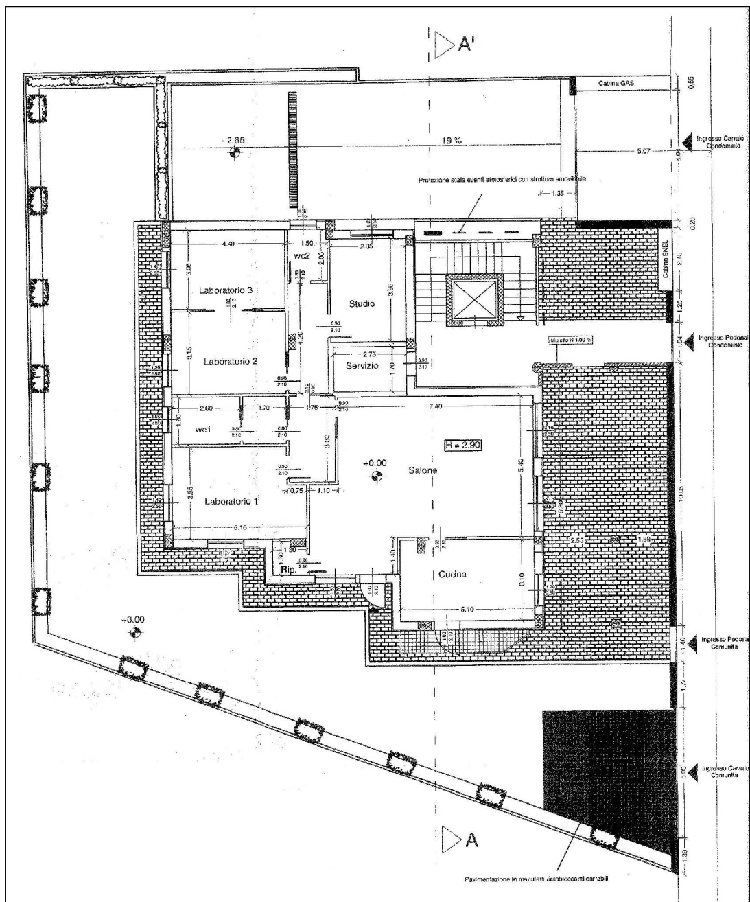
PLANIMETRIA PIANO TERRA SCALA 1:200
