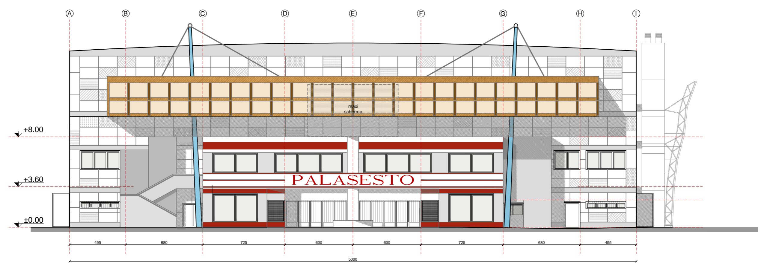
Prospetto Sud-Ovest: Stato di Progetto
